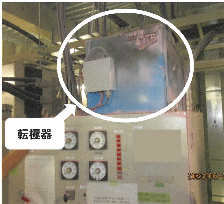
転極器正面
